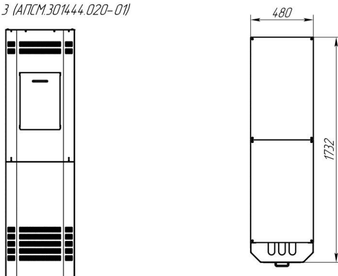
Сборка стеллажа СА-40-120 (МД) с соединением секций по узкой стороне
