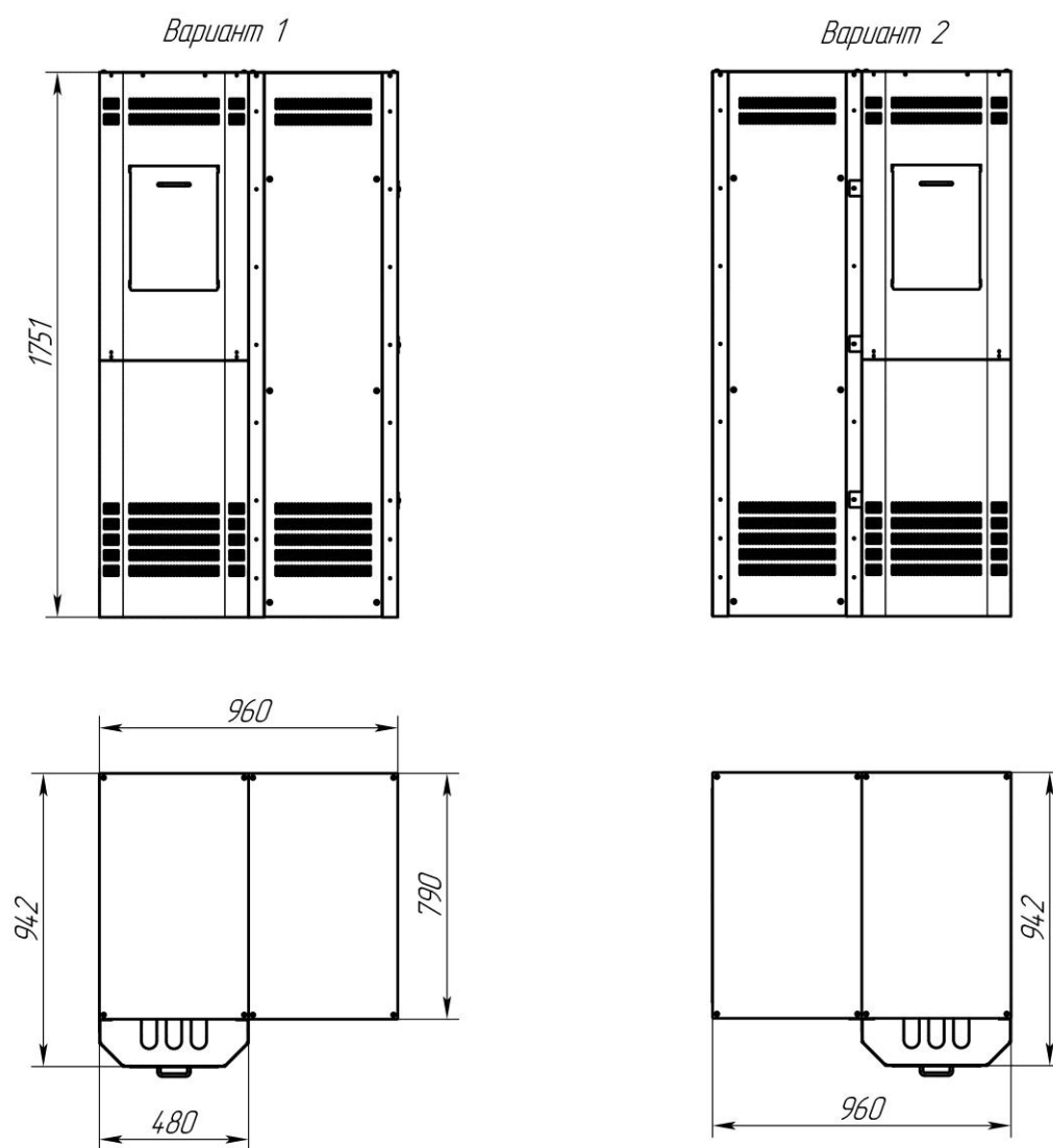
Сборка стеллажа СА-40-120 (МД) с соединением секций по широкой стороне
